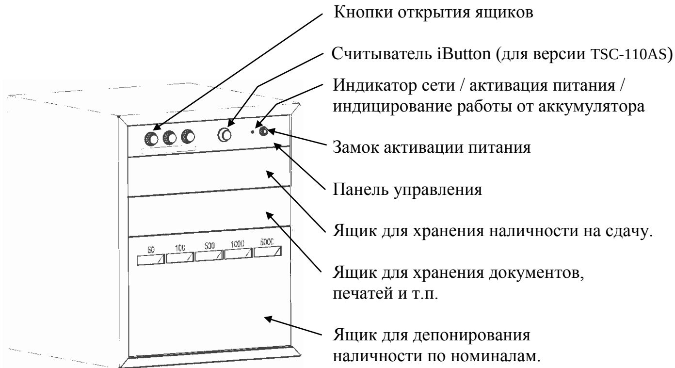
Рис. 1 Общий вид.
